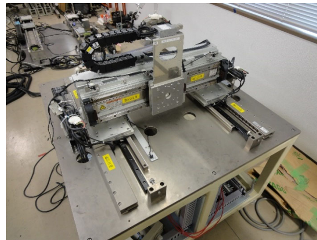
XY軸リニアモータスライダ (Y軸がパラレルツイン機構)
