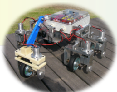
不整地走行ロボット
